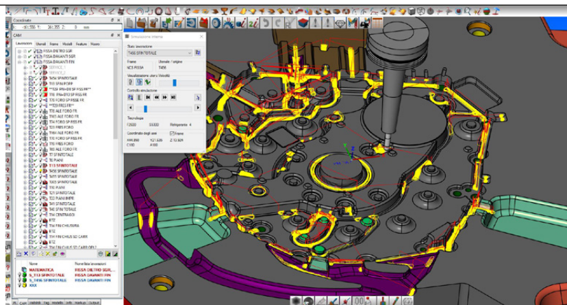
Simulazione lavorazione per corso utensile in hyperMILL
